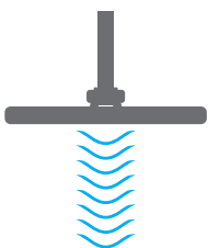
Vista delantera del perfil de señal más intensa usando la bobina Doble D.
